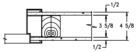
HOISTWAY DOOR STANDARD STEEL STUD CONNECTION
