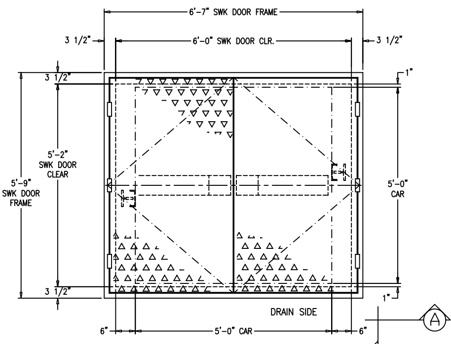
GILCO SIDEWALK DOOR
